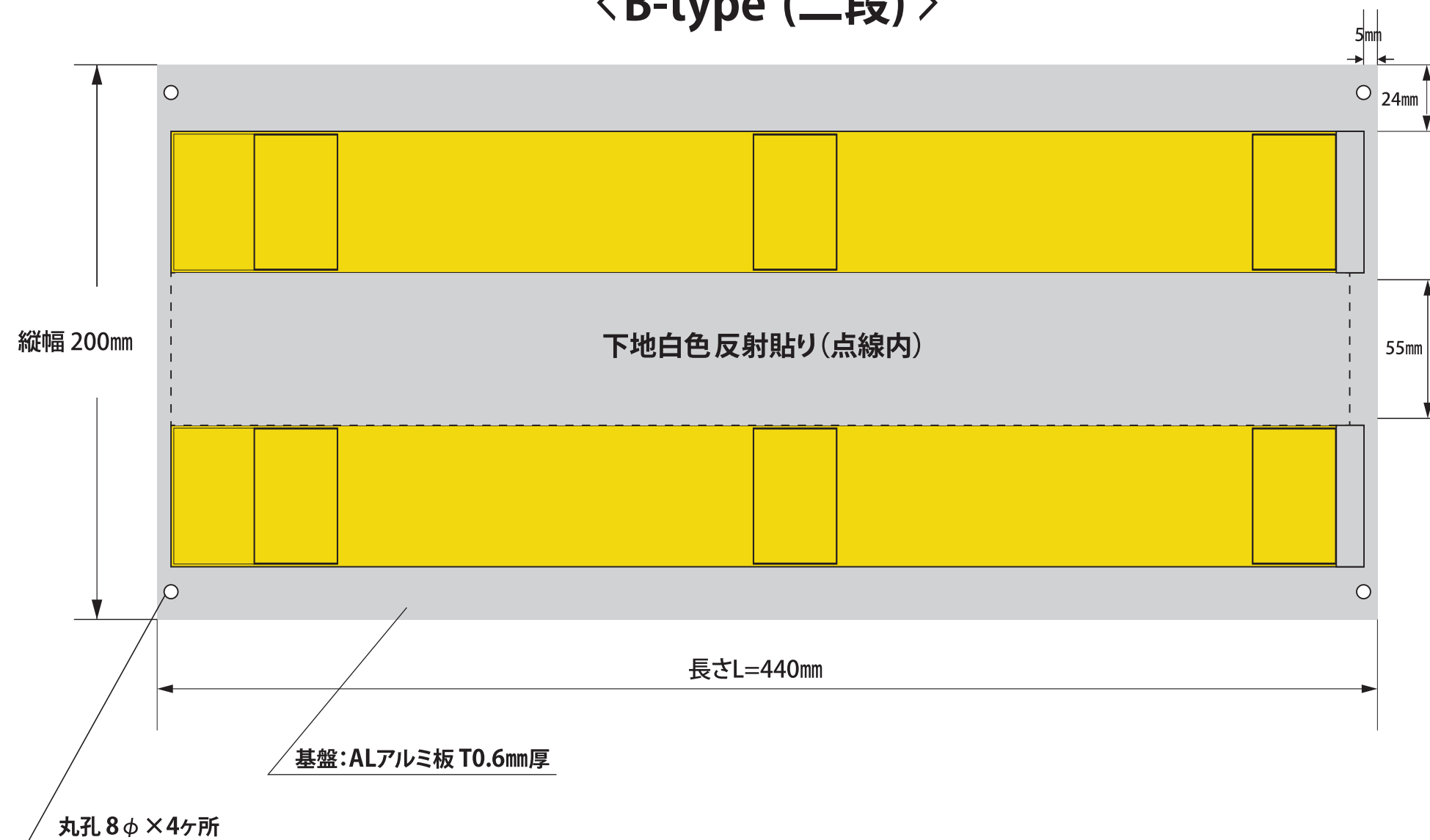
＜B-type (二段)＞
