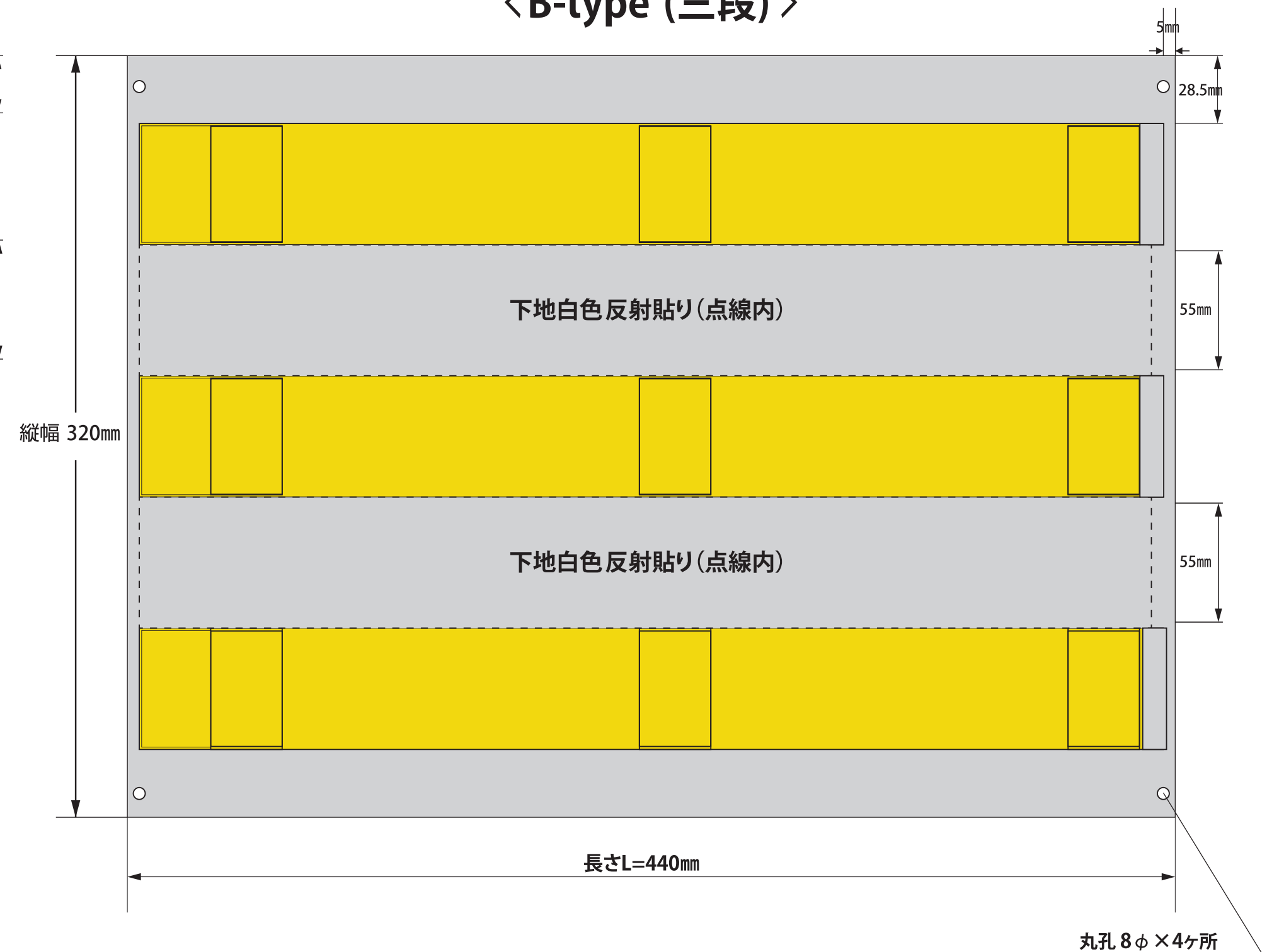
＜B-type (三段)＞
